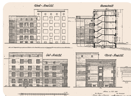
Historische Bauzeichnung Reichardtblock (Foto: altoba)
